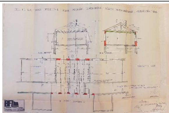
tetőtér újjáépítésének terve
