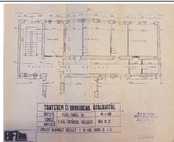
átalakítási tervrajz
