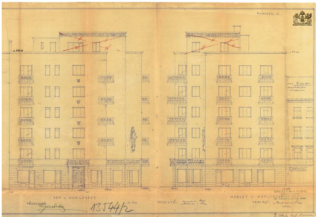
Homlokzati rajzok, 1929 (BFL)
