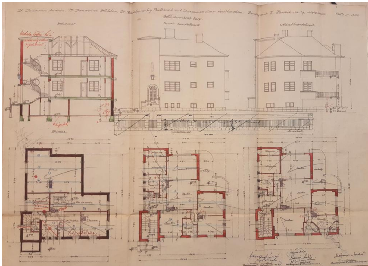
Módosított tervrajzok, 1932 (BLF)
