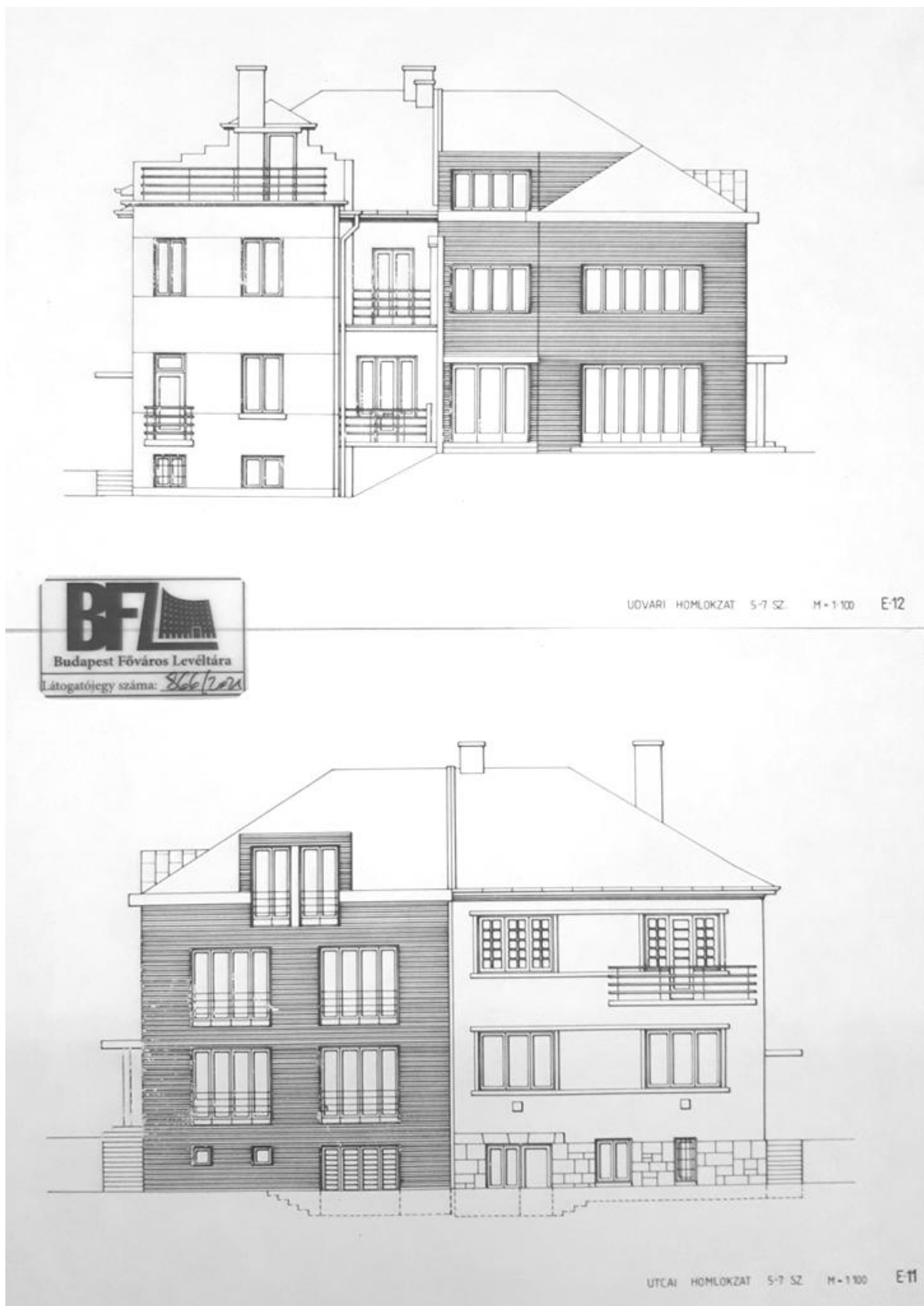
Átalakítási, felújítási tervdokumentáció, 1988 (BFL)
