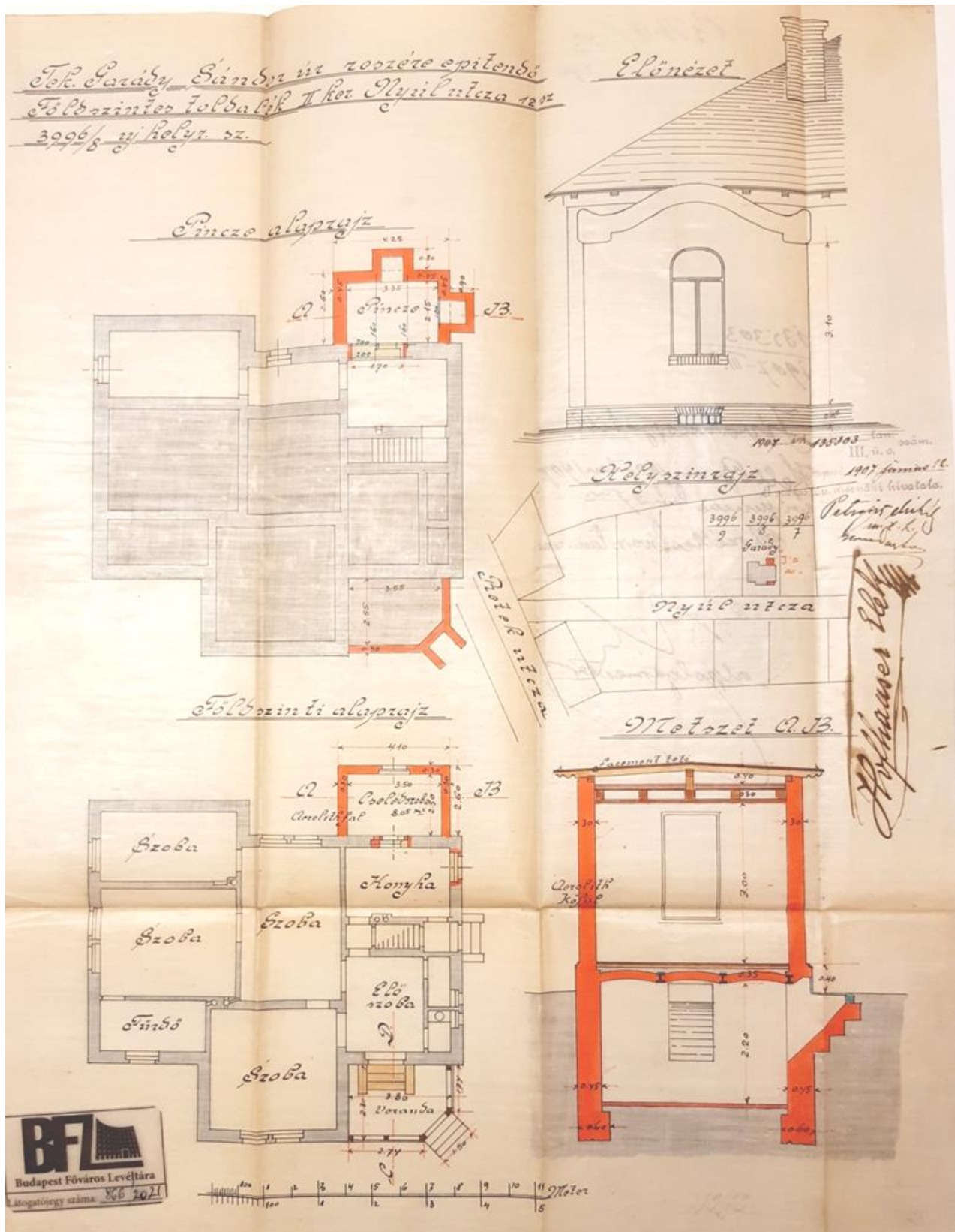
Toldaléképület tervrajzai, 1907 (BFL)
