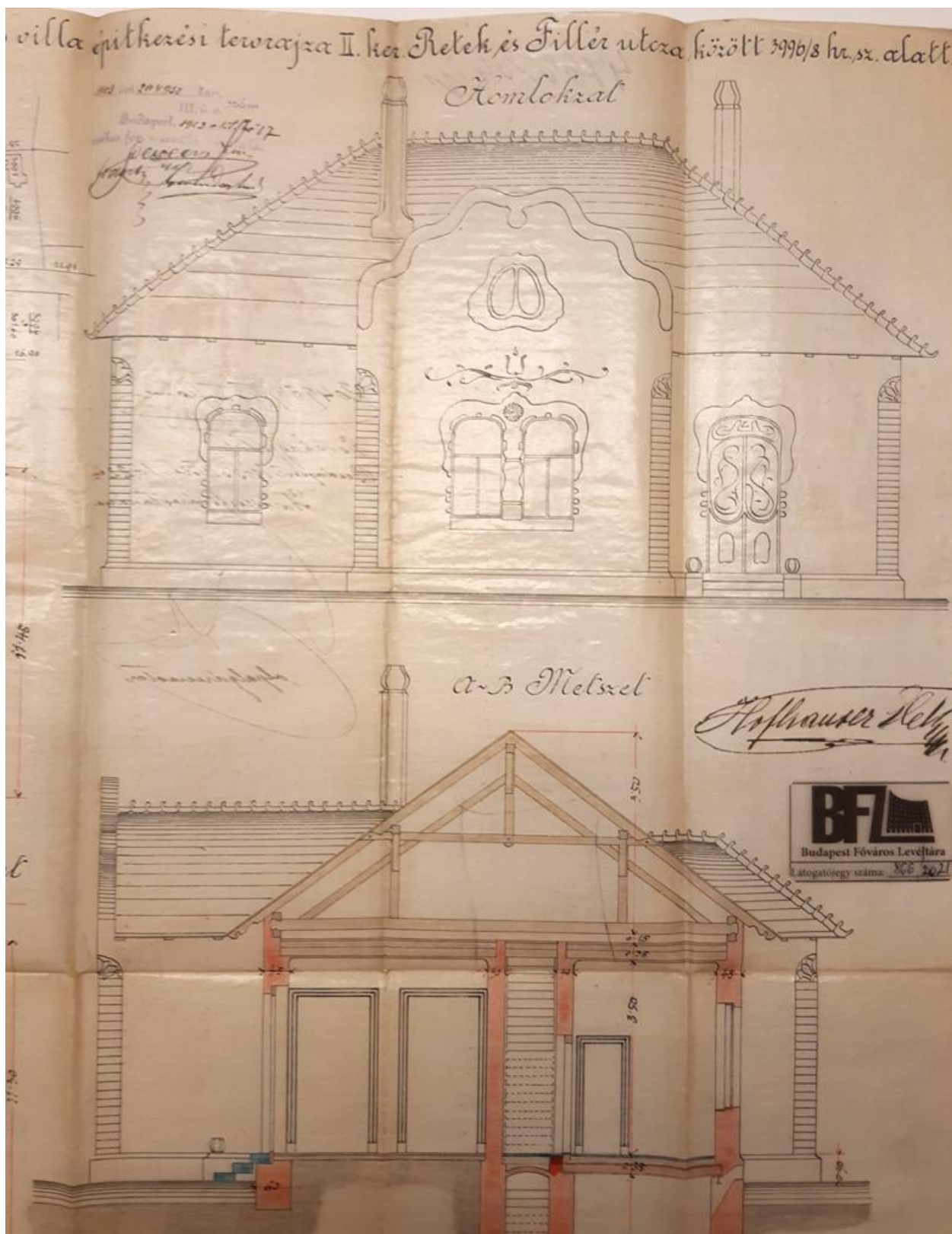
Utcai homlokzat és metszet, 1903 (BFL)
