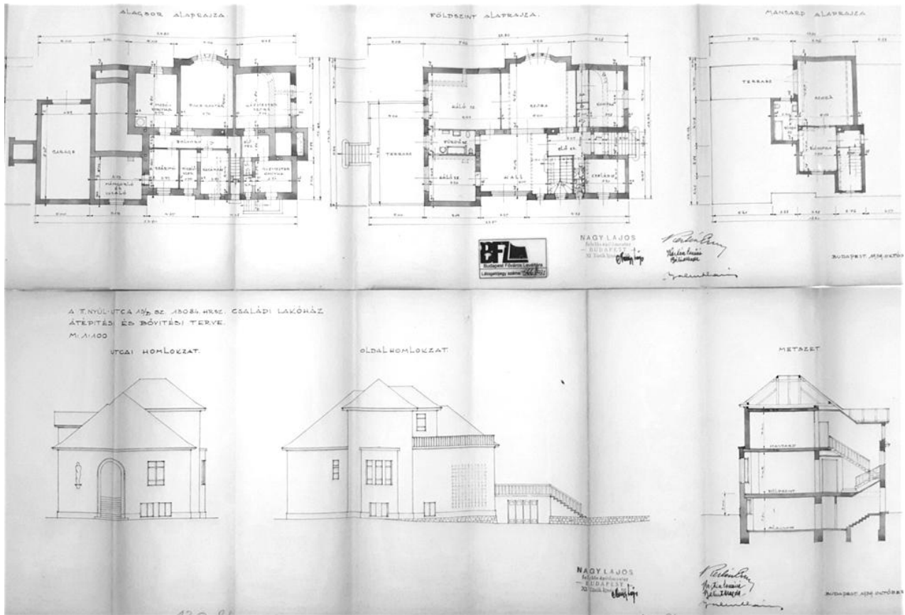
Lakóház átépítés és bővítési terve, 1939 (BFL)
