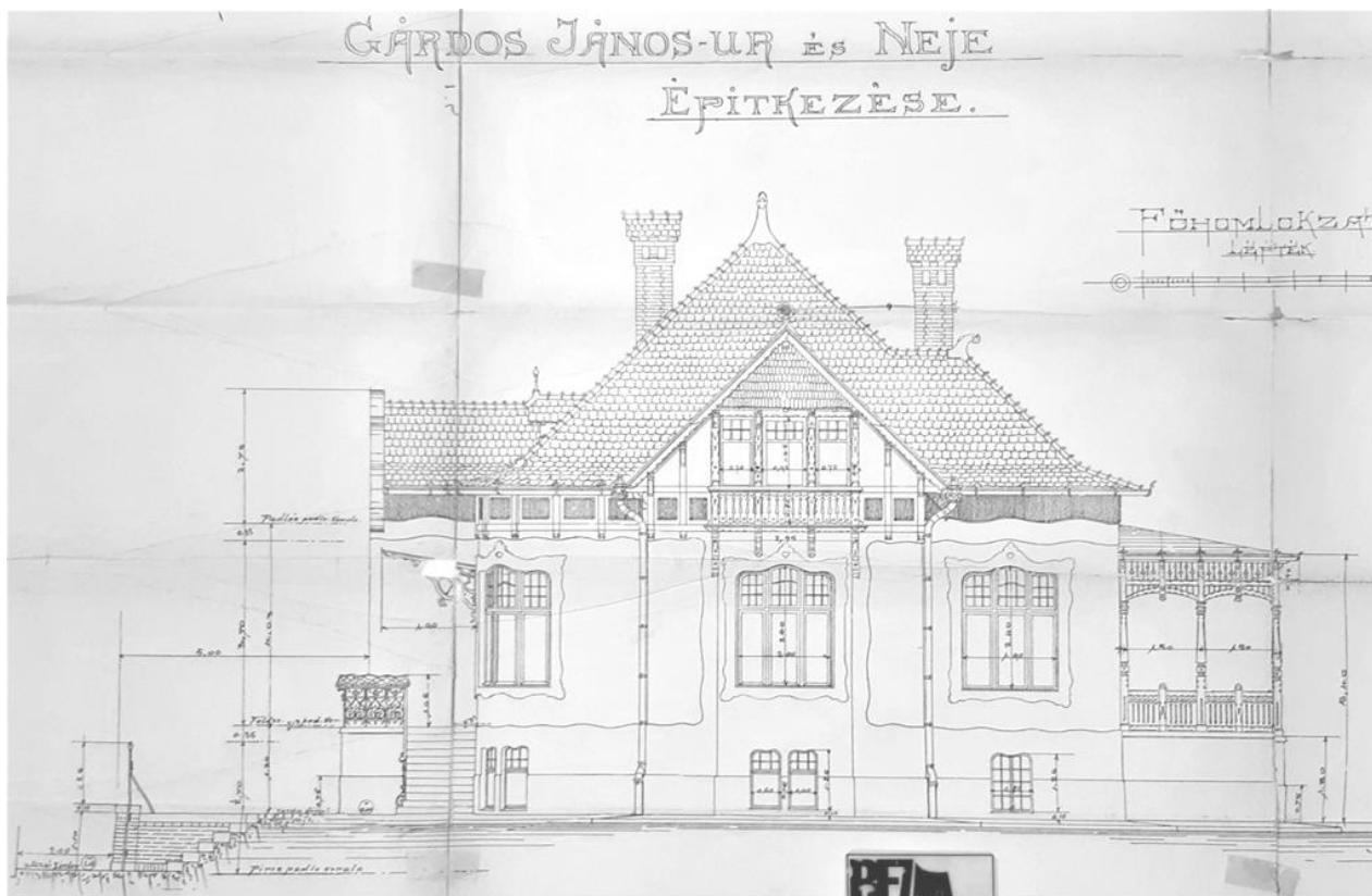
Építési engedély tervrajzai, 1904. (BFL)
