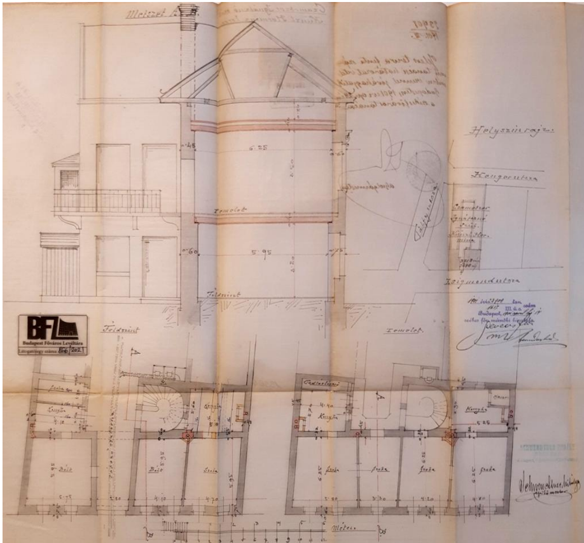
Engedélyezési tervrajz , 1901 (BFL)
