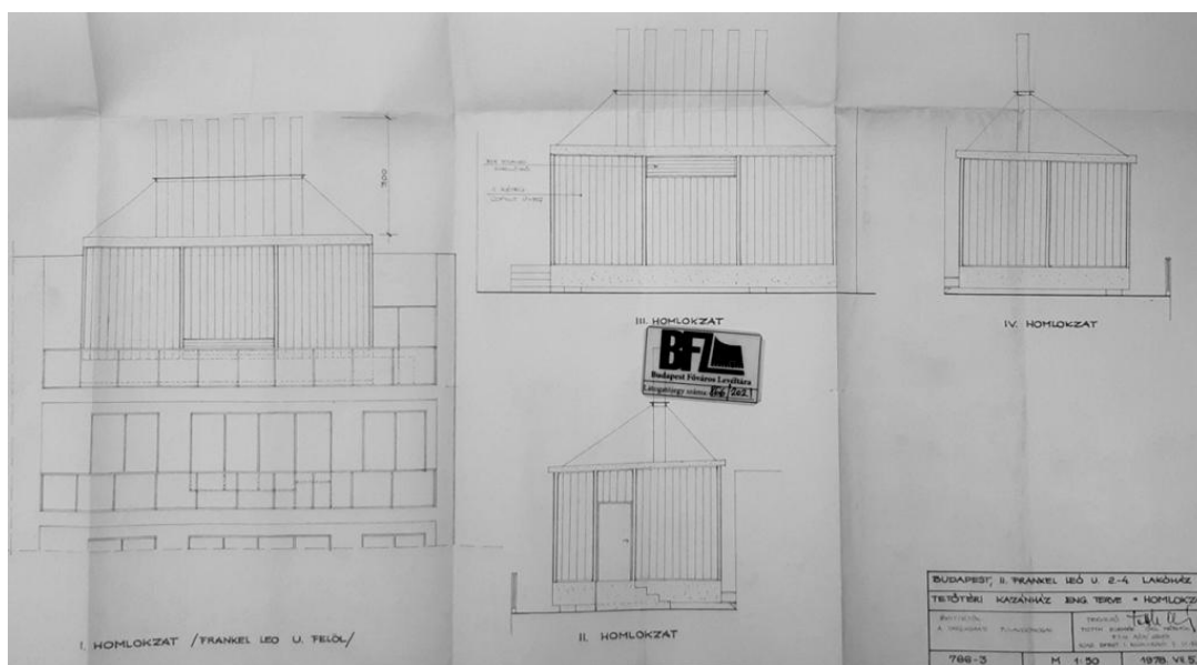
Kazánház engedélyezési terve, 1978 (BFL)
