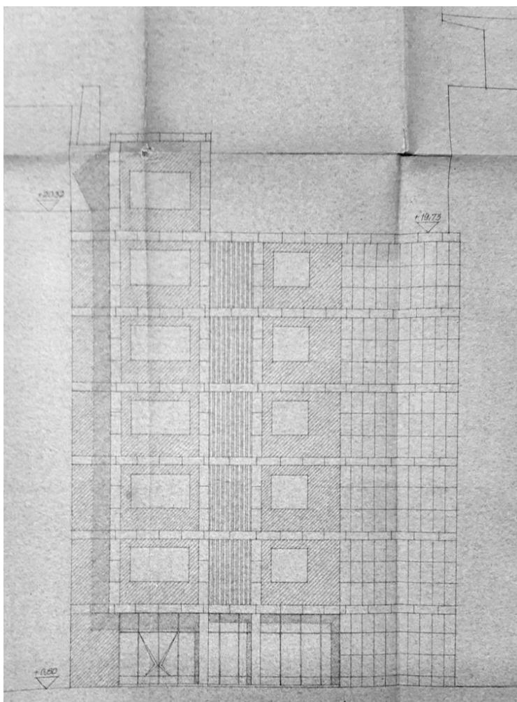
Henger utcai homlokzati rajz, helyszínrajz, 1958 (BFL)
