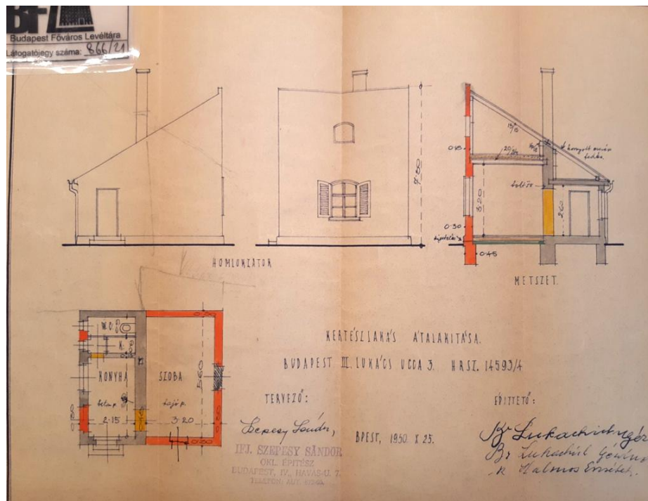
Kertészlakás átalakításának terve, 1950
