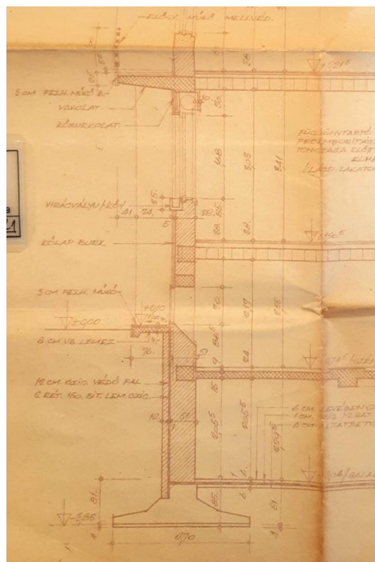
Engedélyezési tervrajzok, 1958 (BFL)
