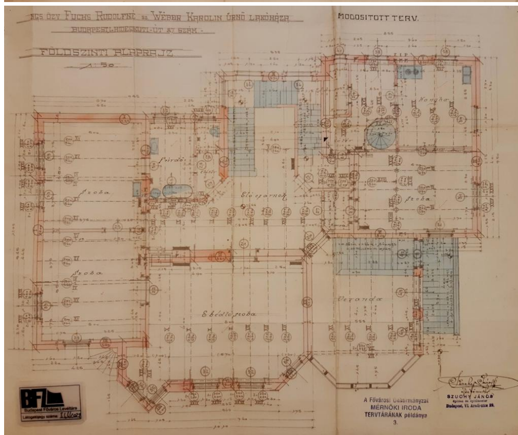
Módosított tervek: szuterén, földszinti alaprajzok, 1910 (BFL)
