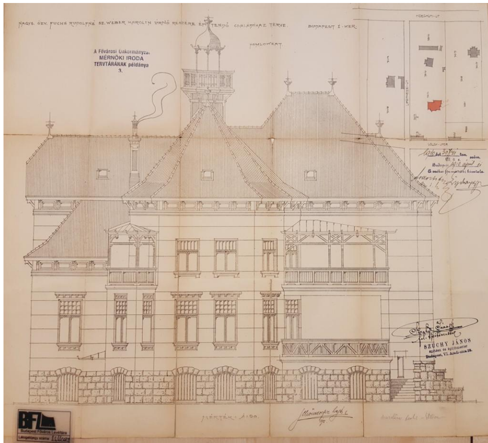
Utcai homlokzat rajza, 1910 (BFL)
