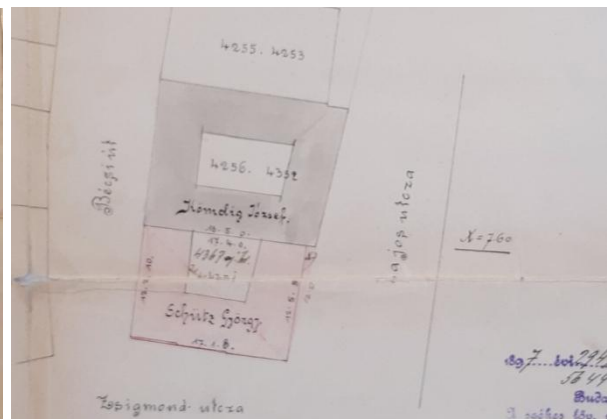
Metszet, alaprajzok, helyszínrajz, 1897 (BFL)
