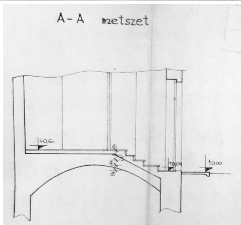
Engedélyezési tervrajzok, 1974 (BFL)
