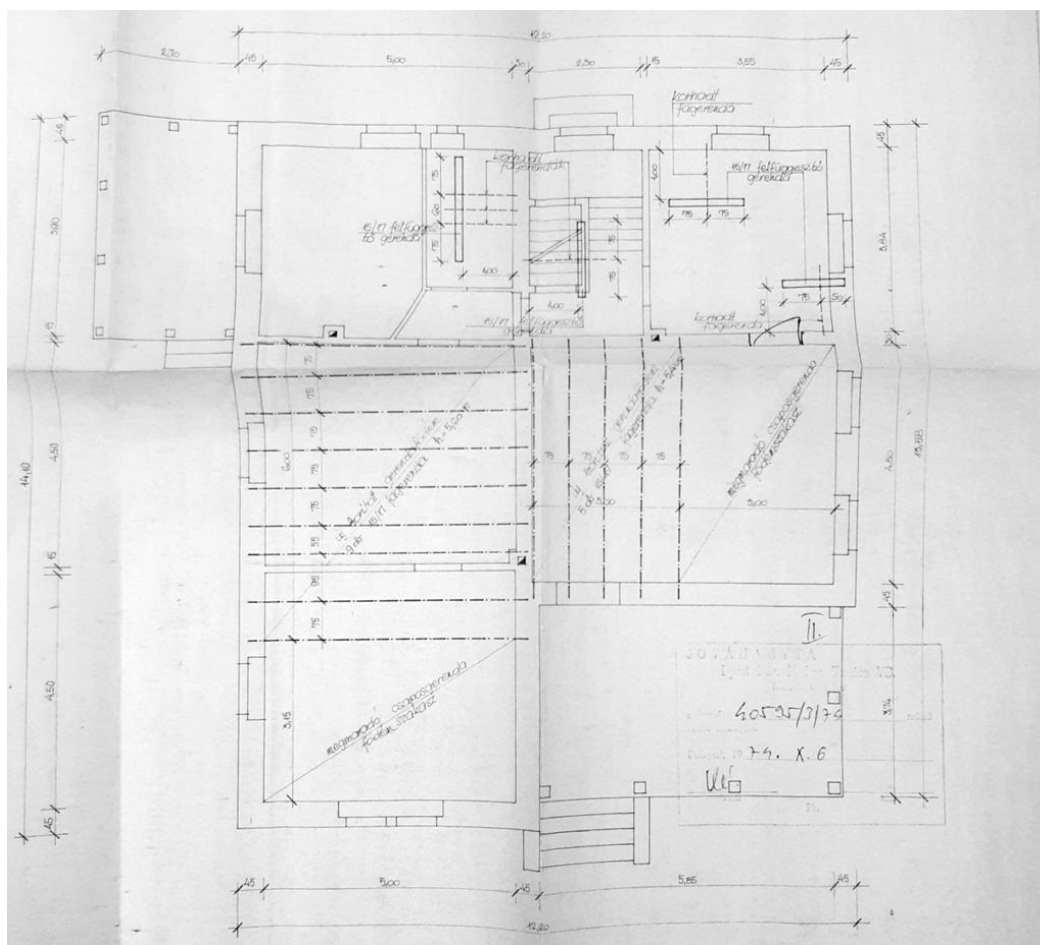
Részleges földemcsere tervrajz, 1974 (BFL)
