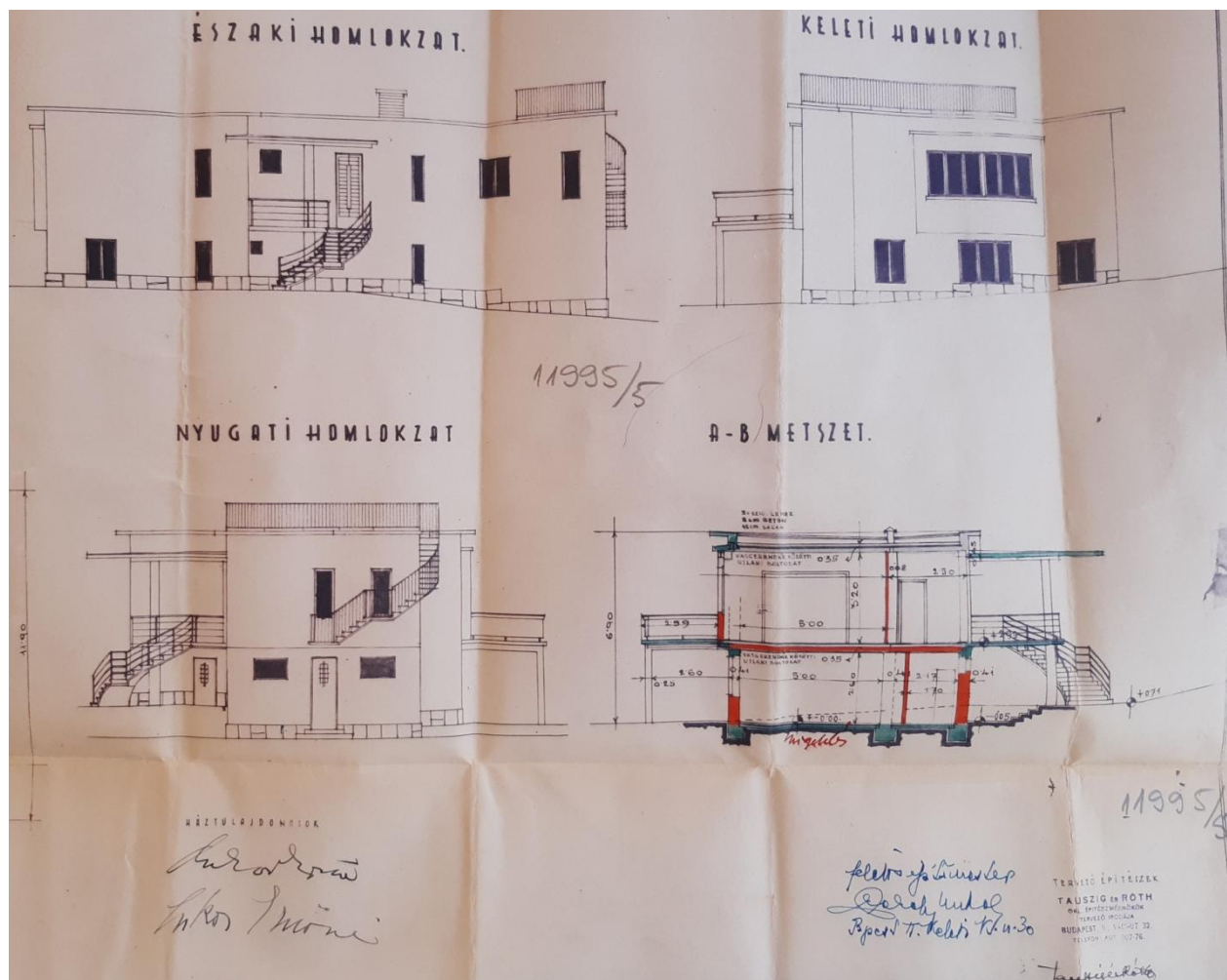
Engedélyezési tervrajzok: homlokzatok, metszet, 1936 (BFL)
