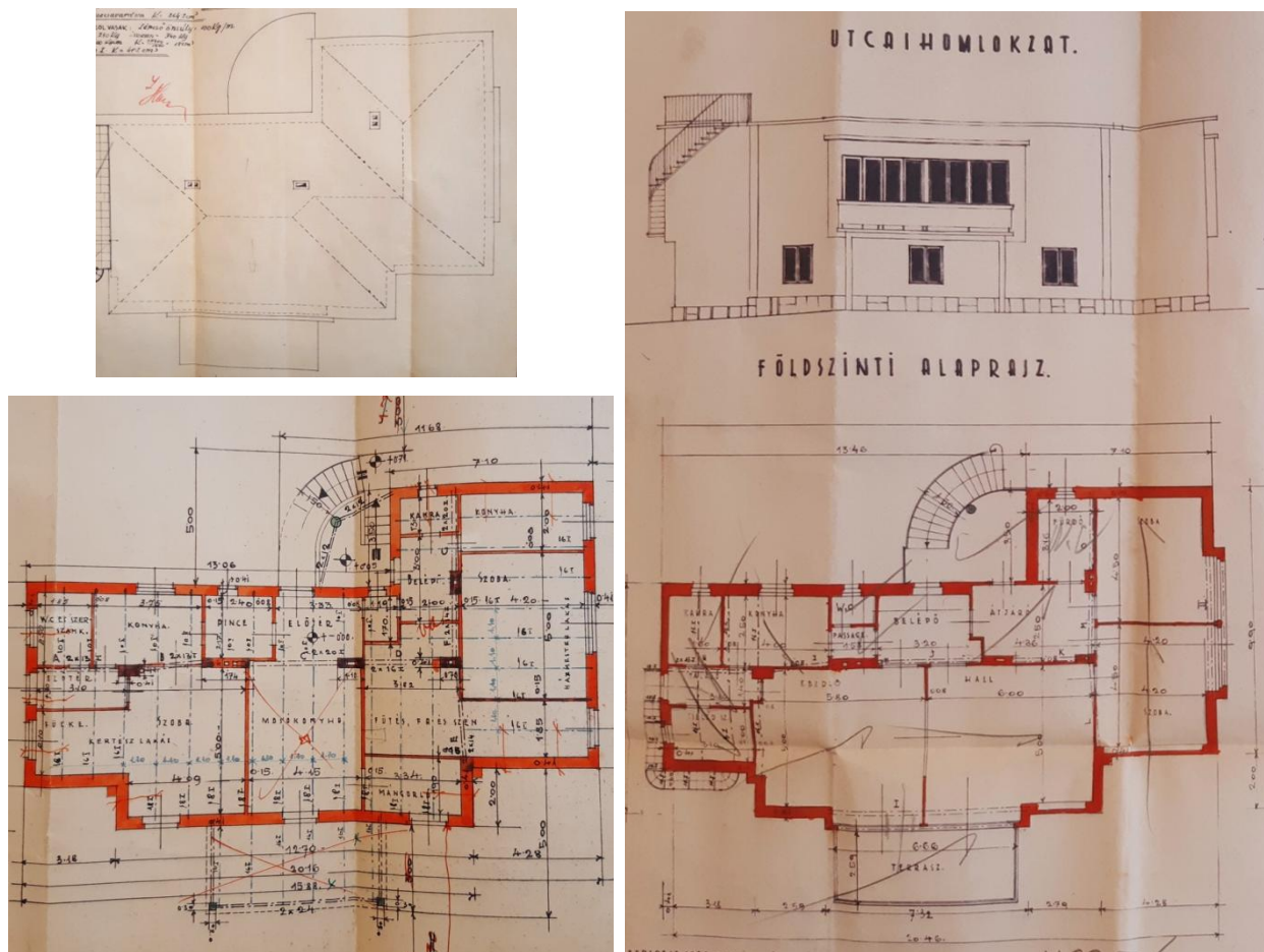
Engedélyezési tervrajzok, 1936 (BFL)
