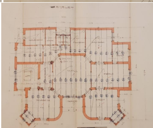
Alaprajzok (souterein, földszint, emelet, padlástér) Metszet, 1910 (BFL)
