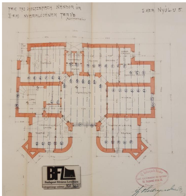
Alaprajzok (souterein, földszint, emelet, padlástér) Metszet, 1910 (BFL)
