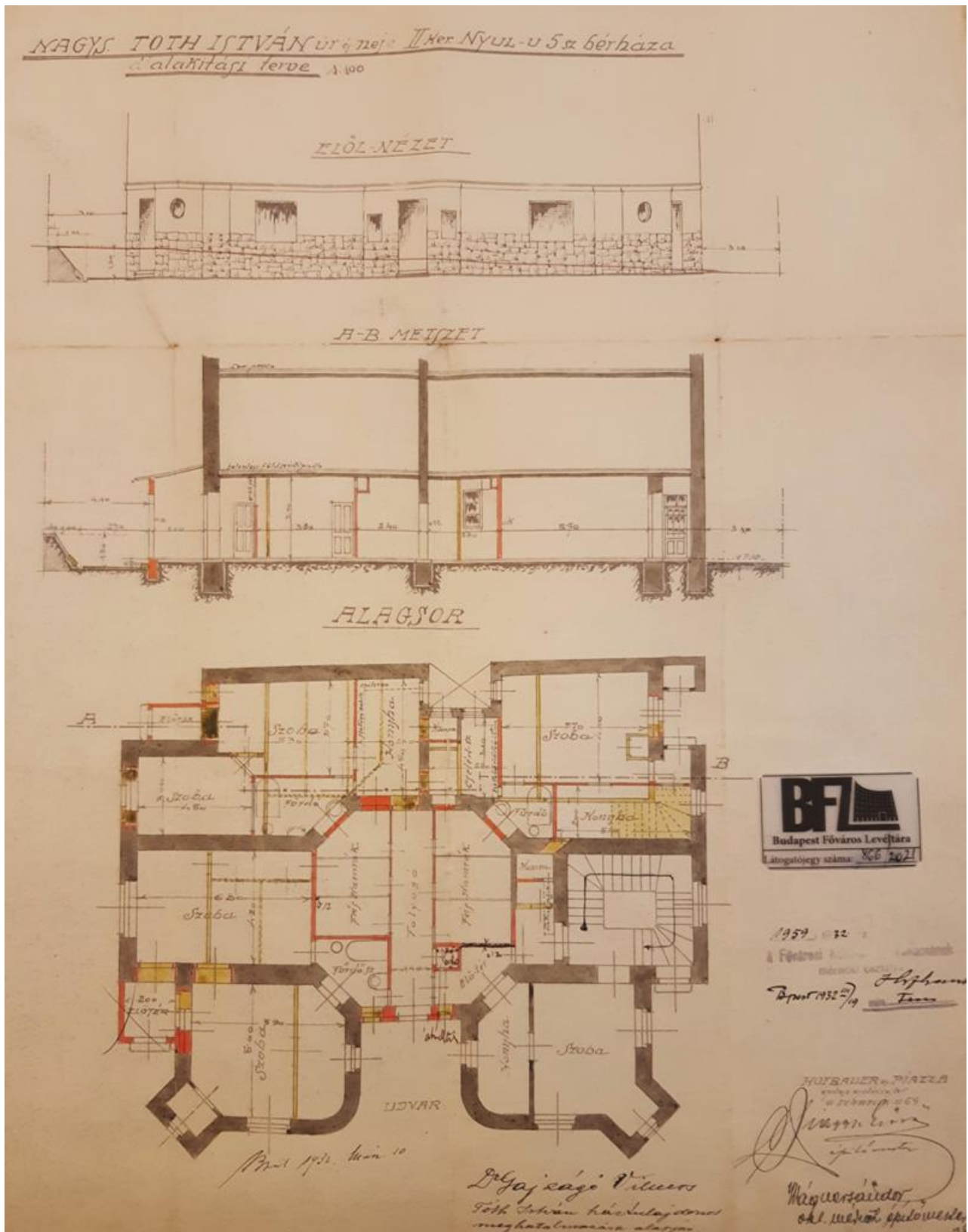
Alagsori alaprajz, 1932 (BFL)
