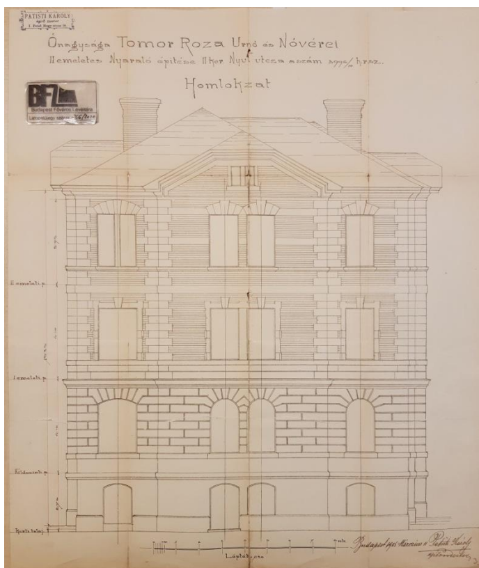
Metszet, homlokzat, 1905 (BFL)
