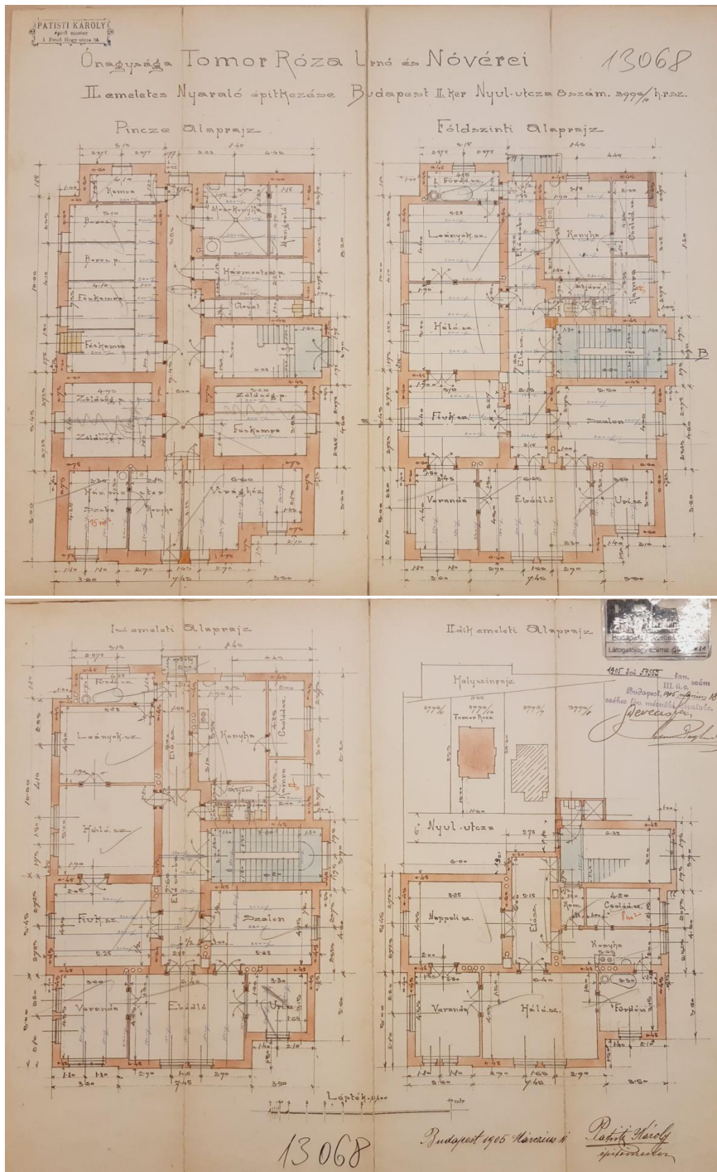
Alaprajzok, 1905 (BFL)
