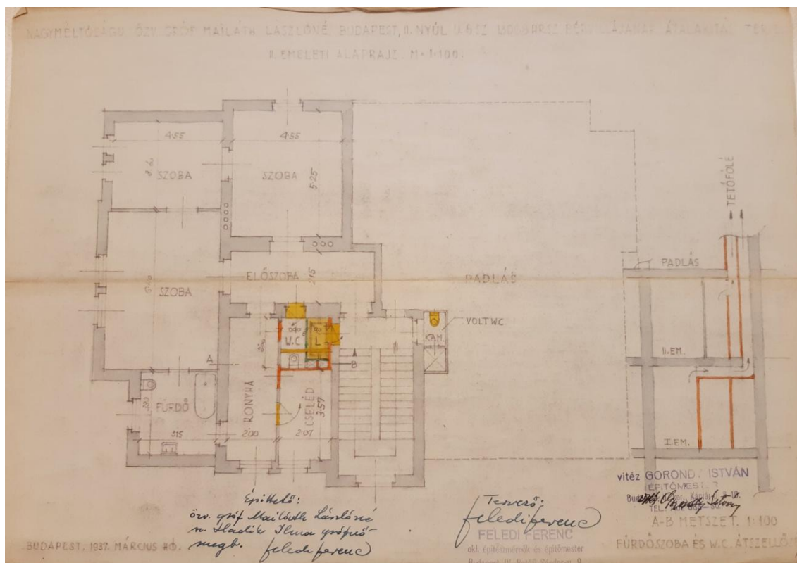
Alaprajz, metszet, 1937 (BFL)
