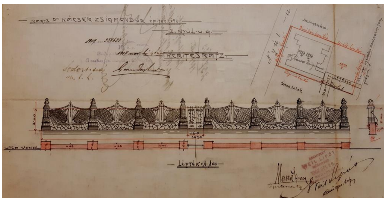
Kerítésrajz, 1907 (BFL)
