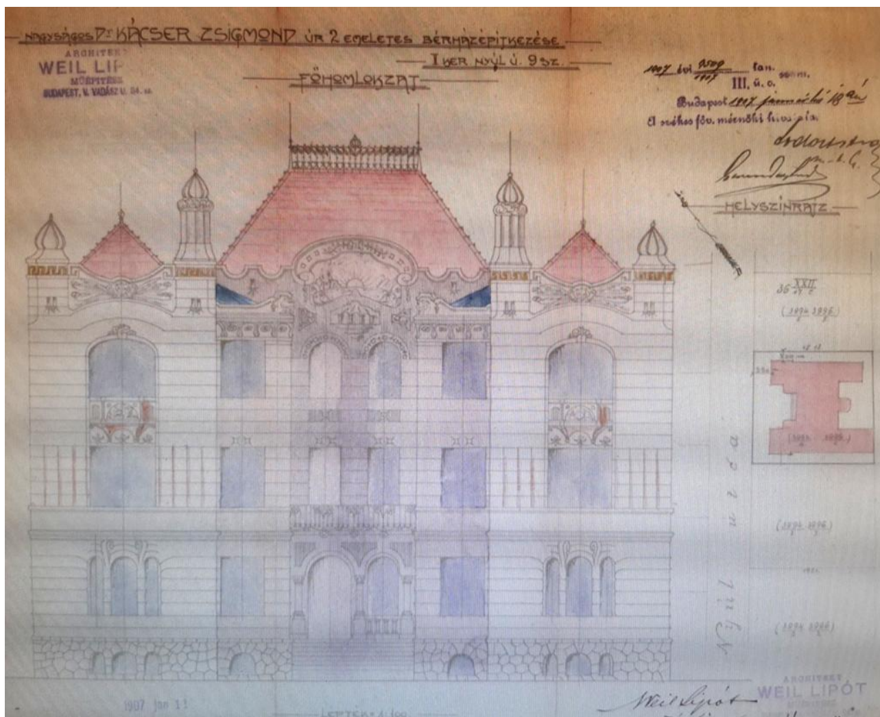
Utcai homlokzat rajza, 1907 (BFL)
