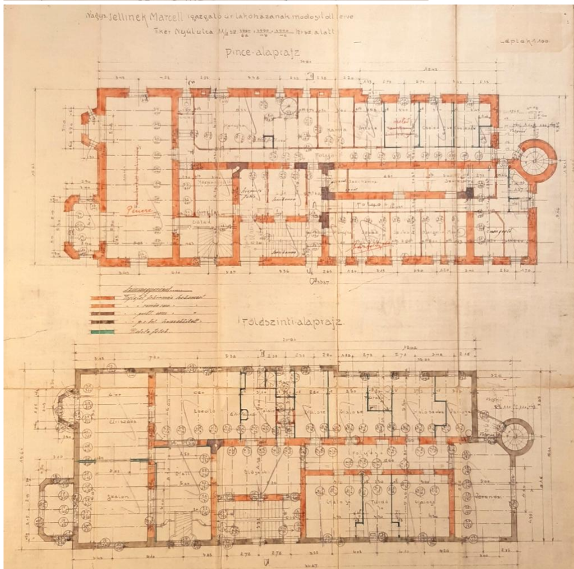
Helyszínrajz, pince, földszint alaprajz, 1911 (BFL)
