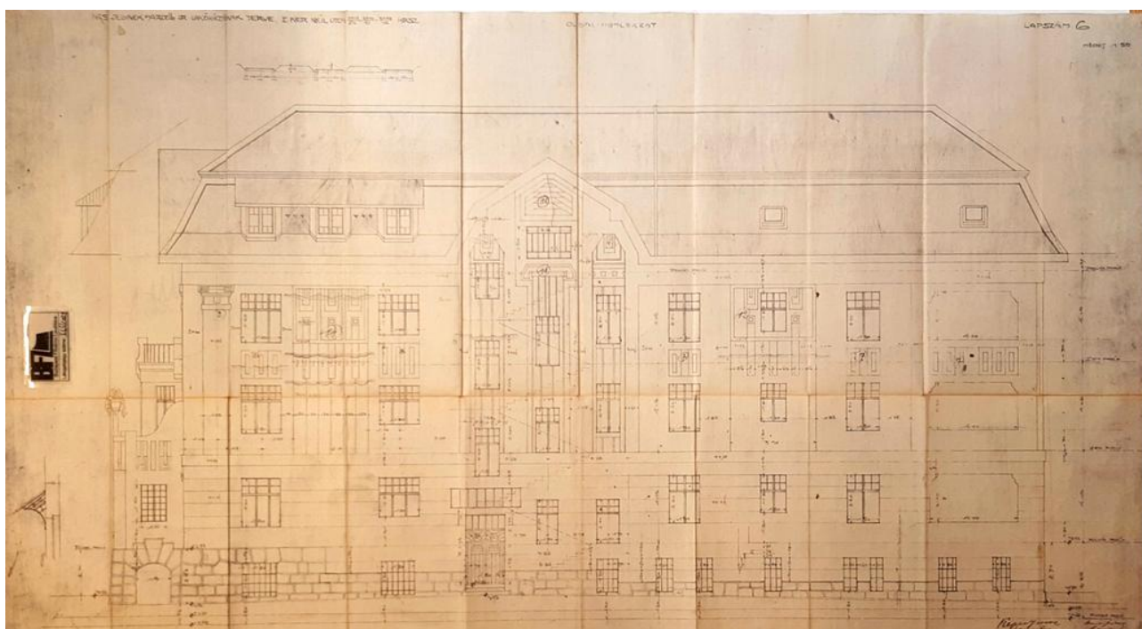
Metszet, homlokzatok, 1911 (BFL)
