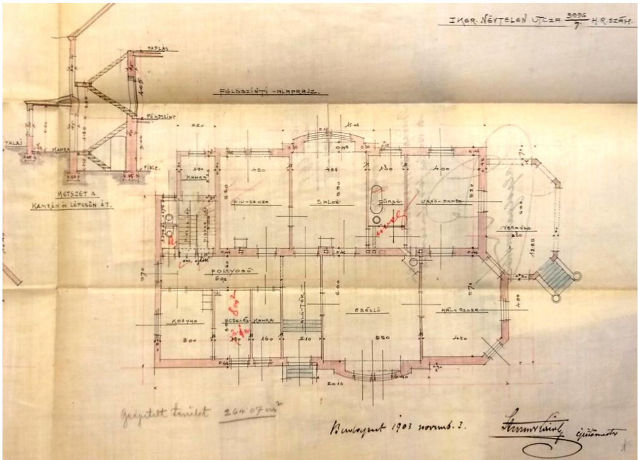
Földszinti alaprajz, 1903 (BFL)
