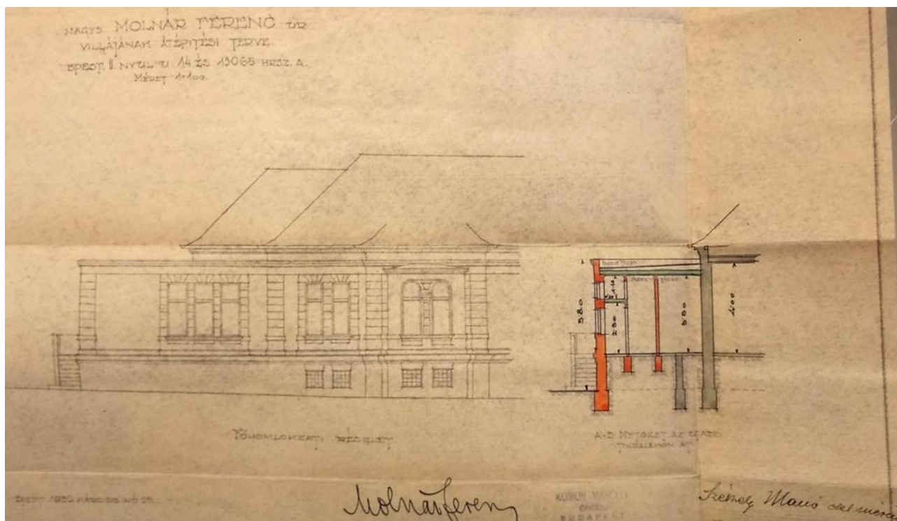
Toldalék építkezés és belső átalakítás: alaprajz homlokzat, metszet, 1932 (BFL)
