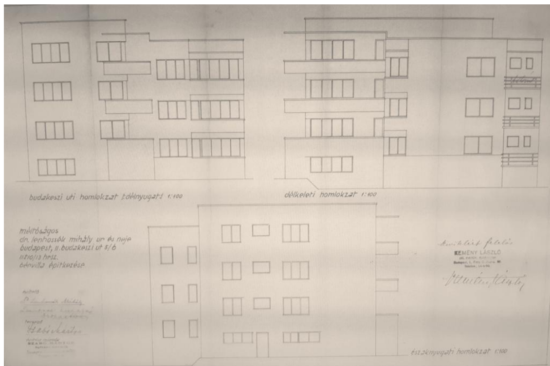
Építési engedély tervrajzai, 1933 (BFL)
