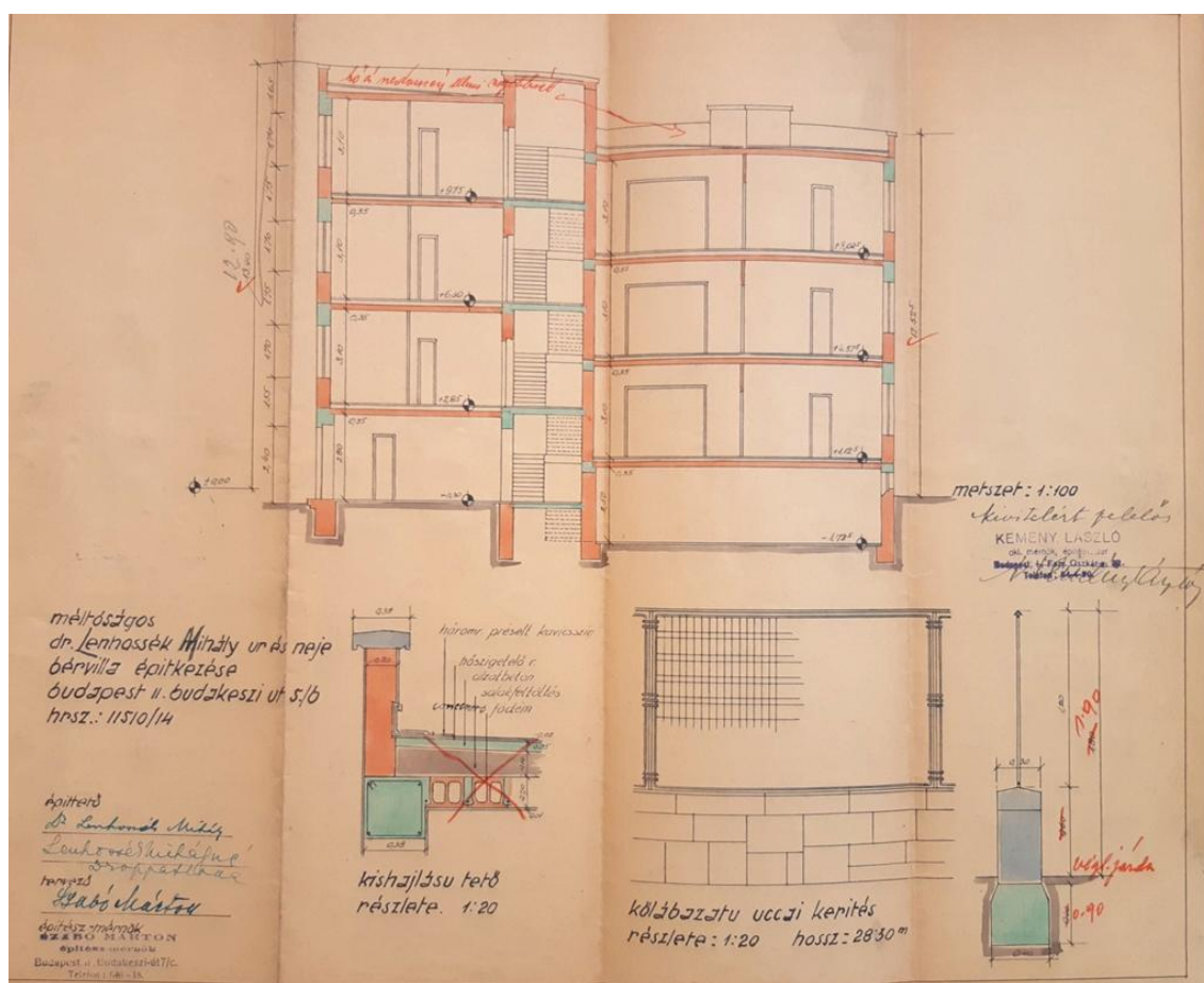
Építési engedély tervrajzai, 1933 (BFL)
