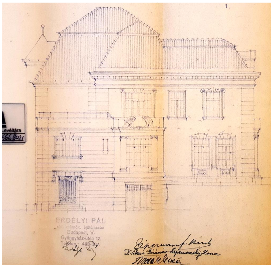
Trombitás utcai homlokzat tervrajza, 1939 (BFL)
