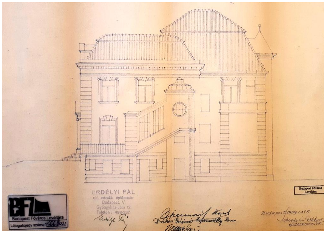
Nyugati (hátsó) homlokzat tervrajza, 1939 (BFL)
