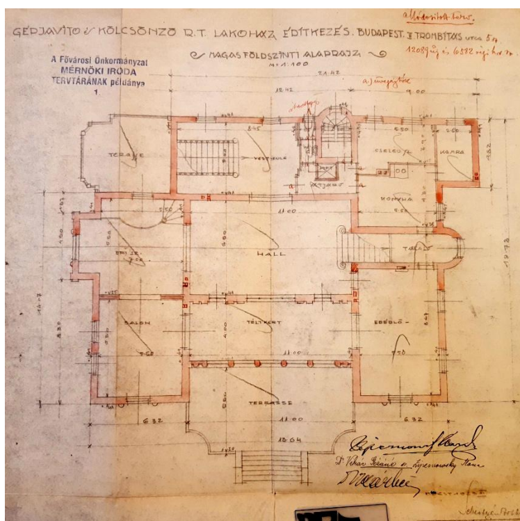
Magasföldszinti alaprajz, 1926 (BFL)
