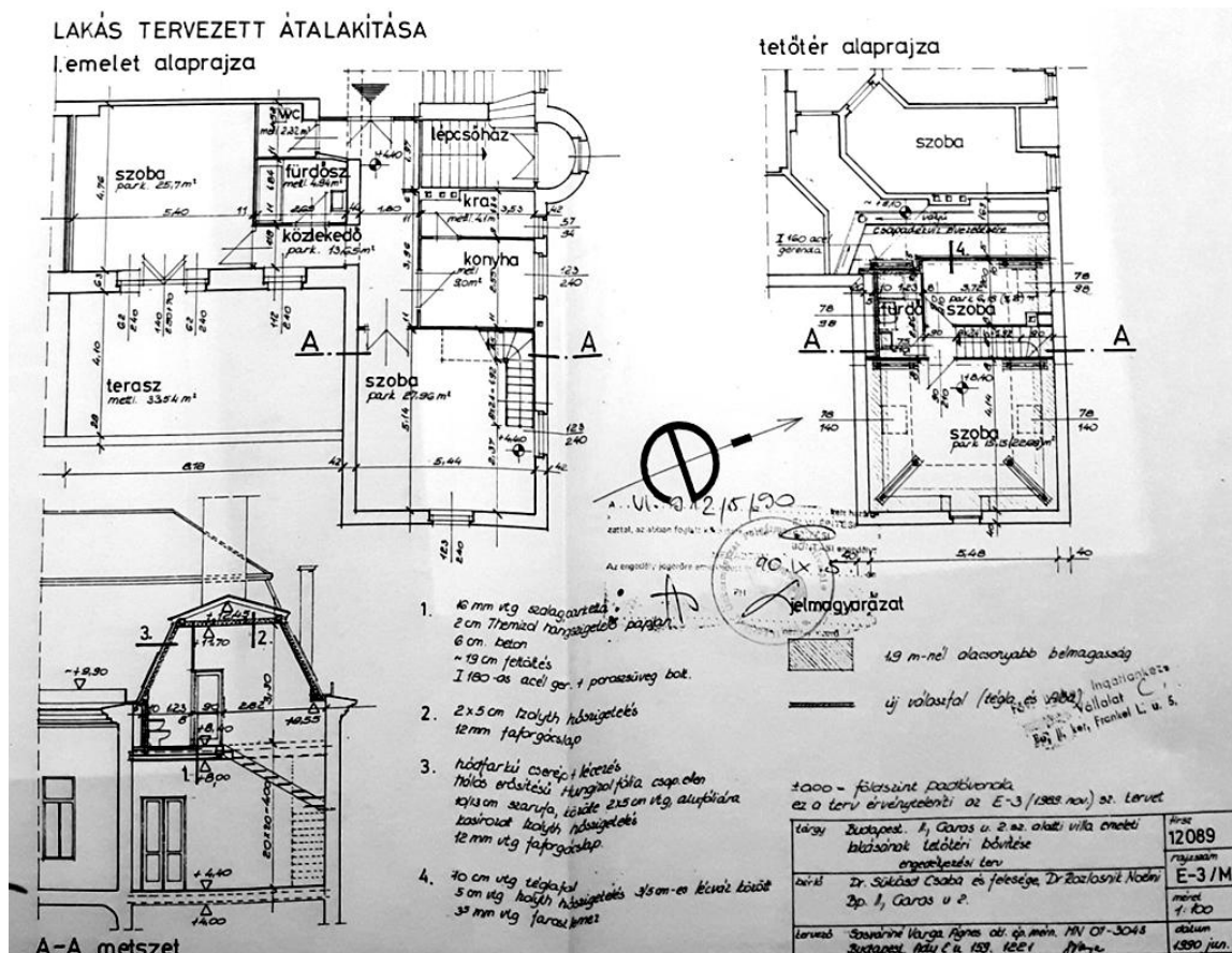
Emeleti lakás tetőtéri bővítése, 1990 (BFL)
