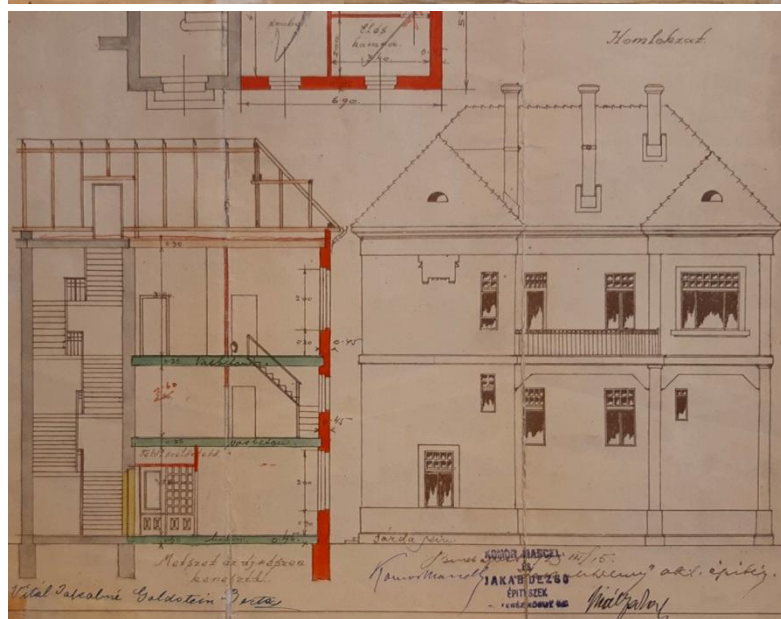
Engedélyezési tervrajzok, 1923 (BFL)
