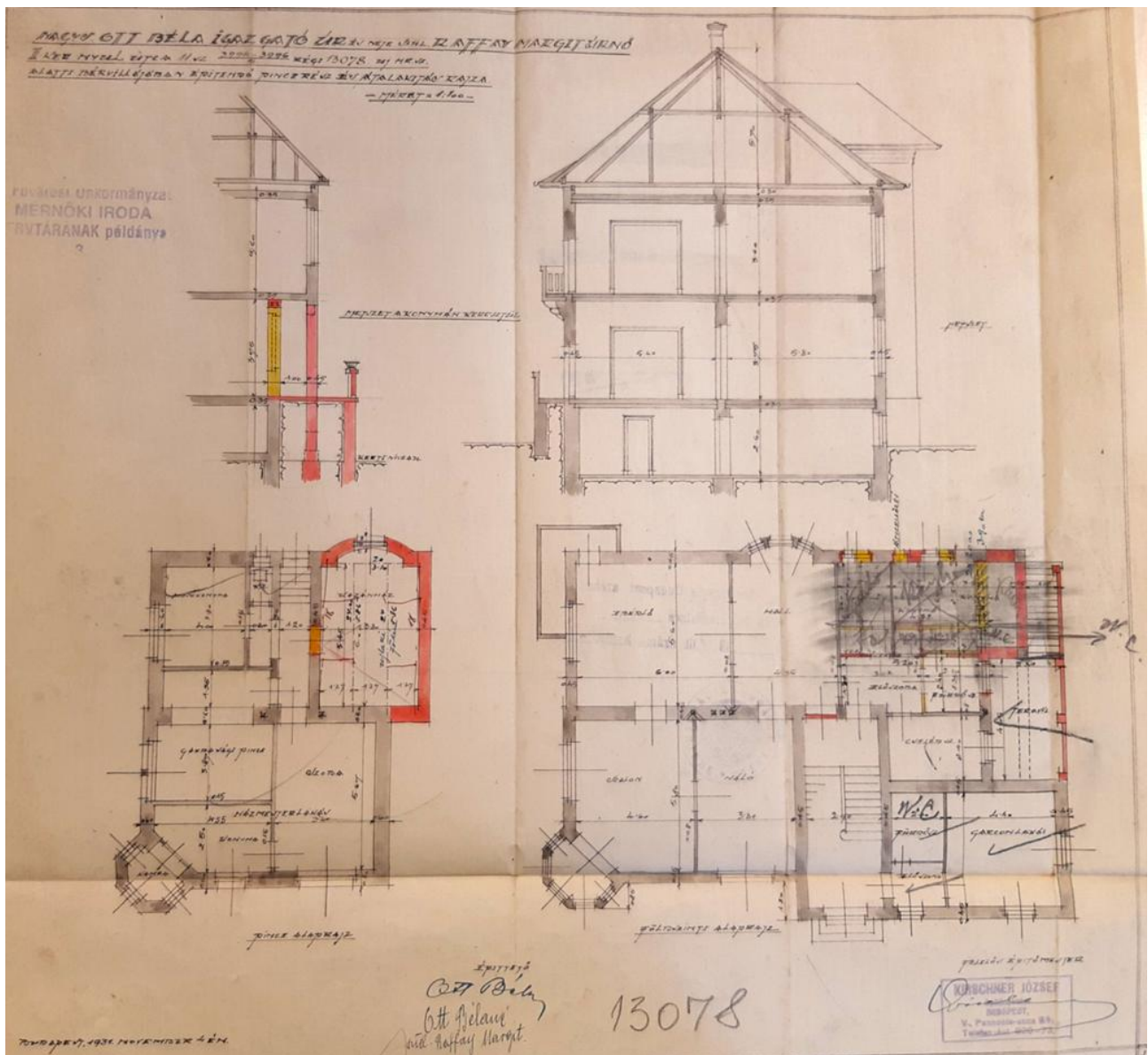
Engedélyezési tervrajz, 1931
