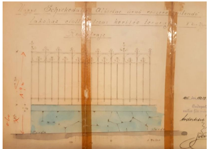
Kerítés részletrajz, 1905
