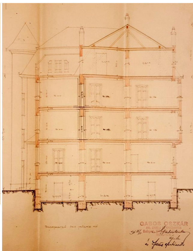
Engedélyezési tervrajzok, 1911 (BFL)
