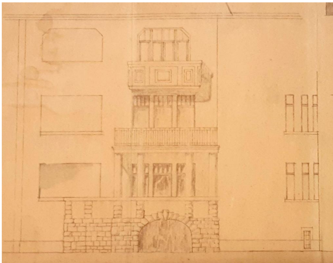
Első emeleti erkély építése - tervdrajzok, 1913 (BFL)
