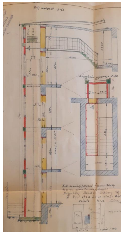
Garázs és személyfelvonó engedélyezési tervrajz, 1939 (BFL)
