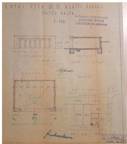
Garázs engedélyezési tervrajz, 1937 (BFL)
