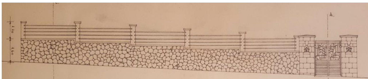
Engedélyezési tervrajzok, 1928 (BFL)
