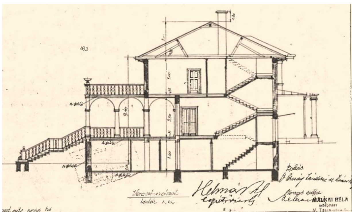
Engedélyezési tervrajzok: nyugati, déli homlokzatok, metszet 1931 (BFL)
