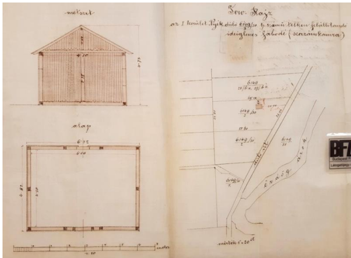
Engedélyezési terv, 1897 (BFL)
