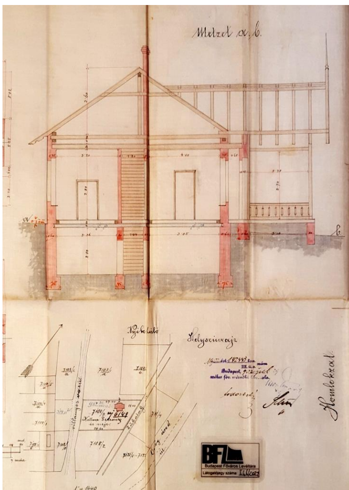
Engedélyezési tervrajzok, 1902 (BFL)
