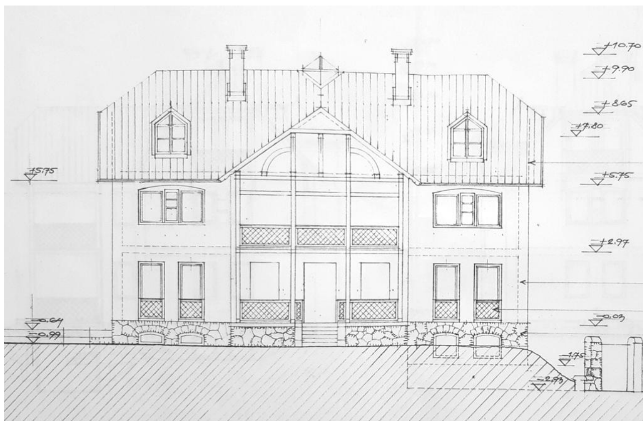
Engedélyezési terv, dél-keleti homlokzat, 1987 (BFL)
