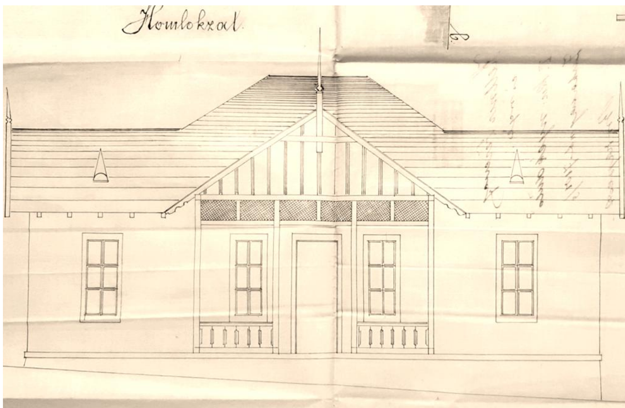
Engedélyezési terv, dél-keleti homlokzat, 1902 (BFL)
