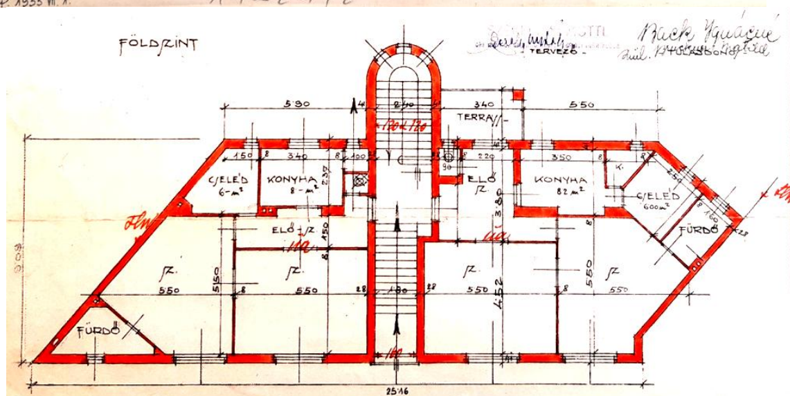
Engedélyezési tervrajzok, 1933 (BFL)
