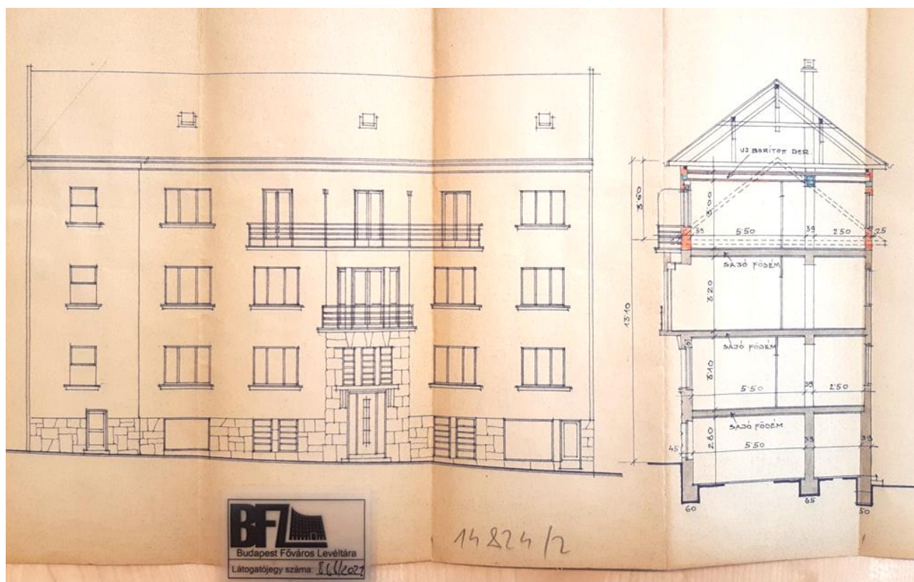
Engedélyezési tervrajz – utcai homlokzat, 1943 (BFL)
