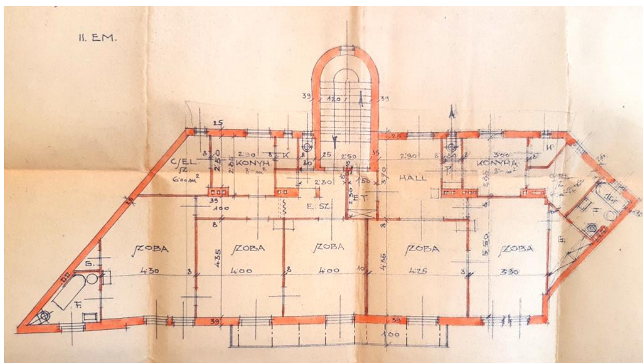
Engedélyezési tervrajz - 2.emeleti alaprajz, 1943 (BFL)
