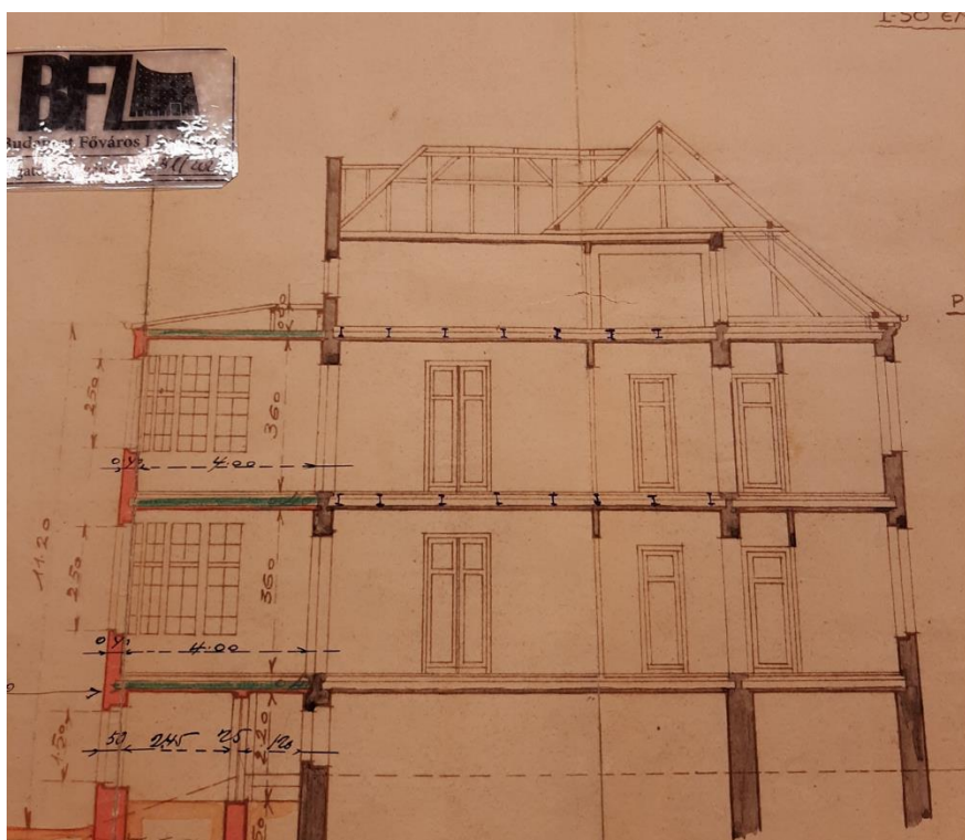
Metszet (1923 BFL)
