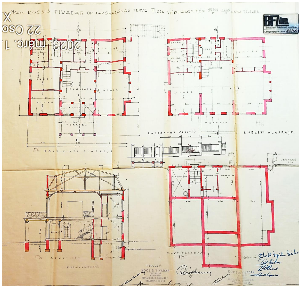
Kocsis-villa alaprajz, Budapest, 1936 (BFL)
