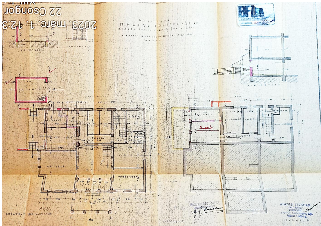
Magyar Posztógyár tulajdonában álló Kocsis-villa átalakítási tervrajza, Budapest, 1938 (BFL)
