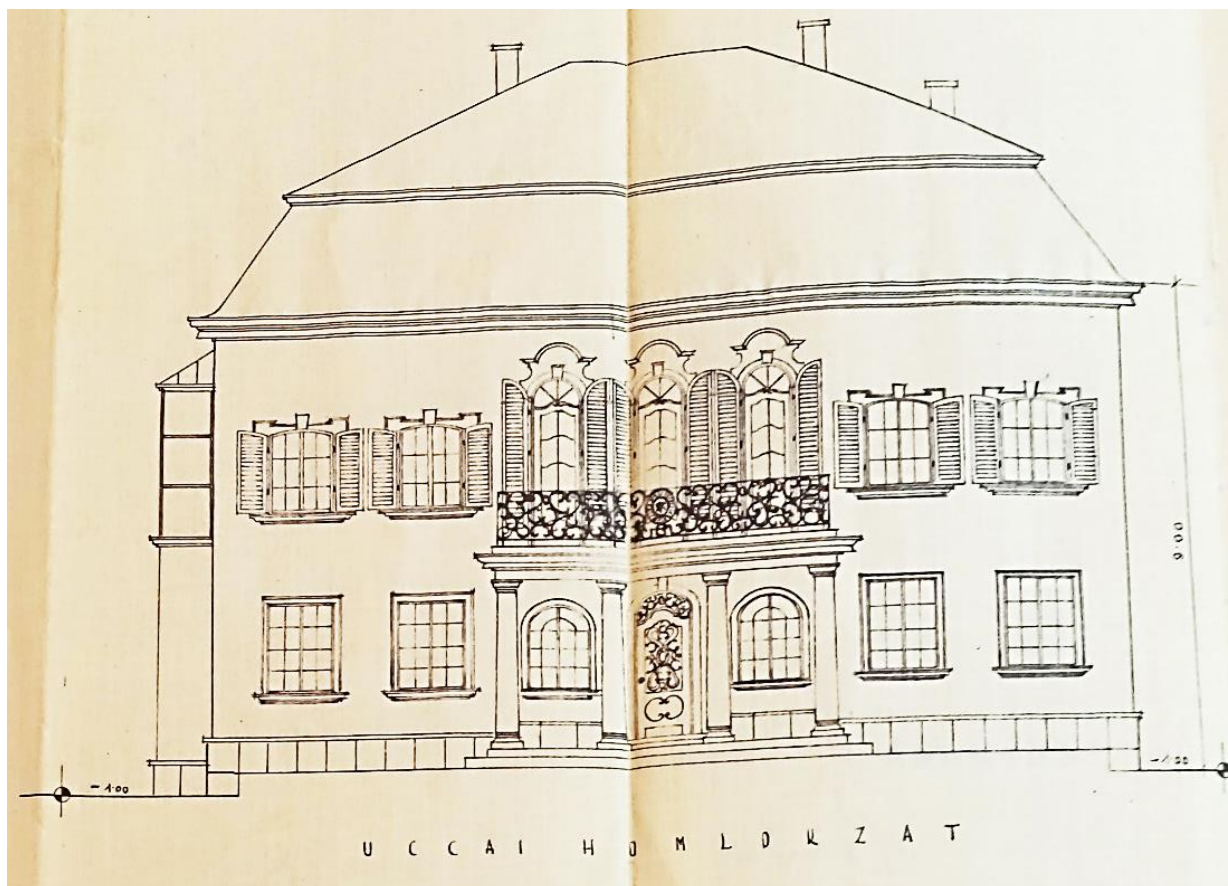
Kocsis-villa utcafronti homlokzat módosított tervrajz, Budapest, 1936 (BFL)
