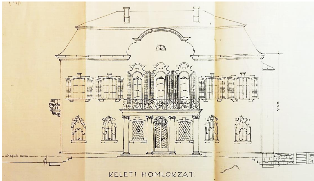
Kocsis-villa utcafronti homlokzat tervrajz, Budapest, 1936 (BFL)
