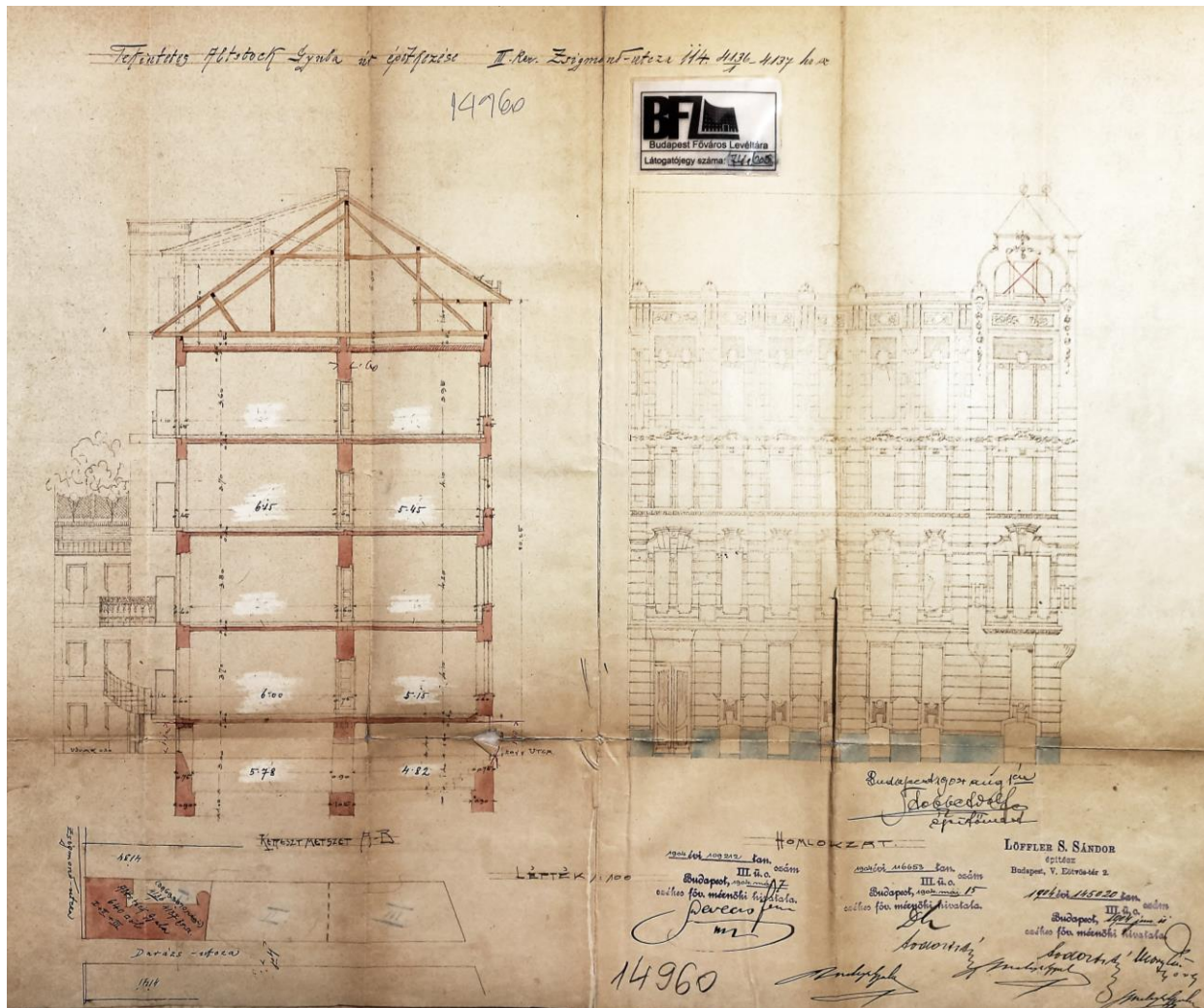
Metszeti és homlokzati tervrajz, 1904, Budapest (BFL)
