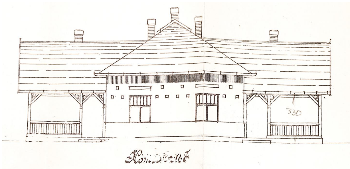
Utcai homlokzat, 1909 (BFL)
