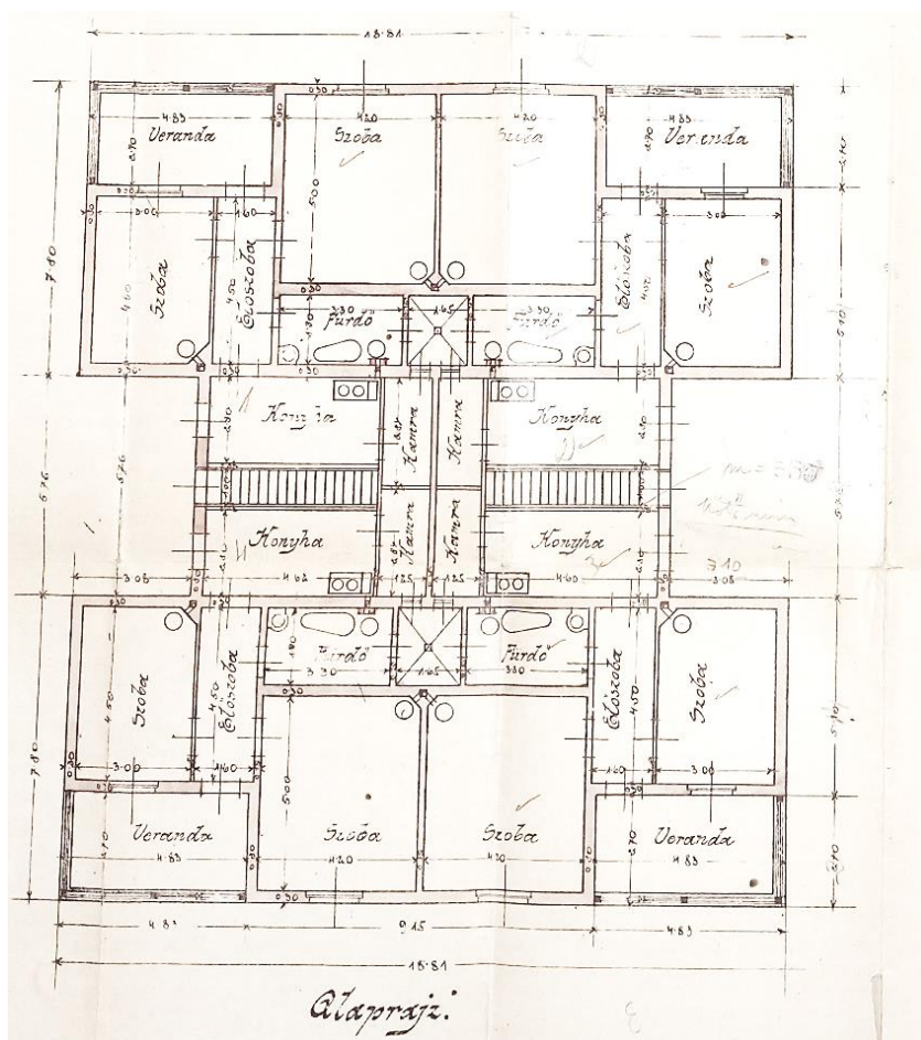
Földszint alaprajz, 1909 (BFL)
